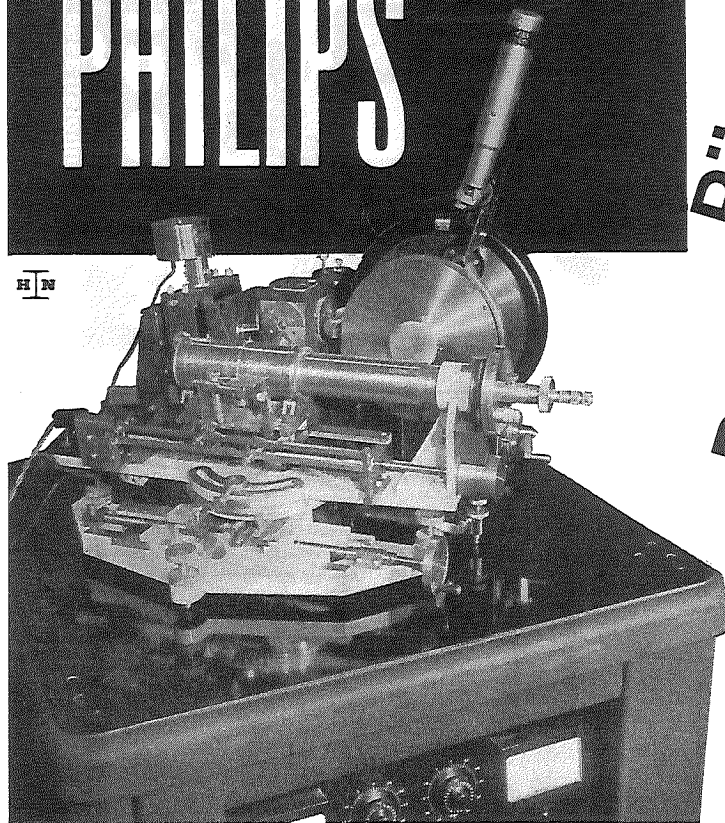
Stabilisierter Röntgenapparat Typ PW 1010 mit Kamera und Goniometer.
