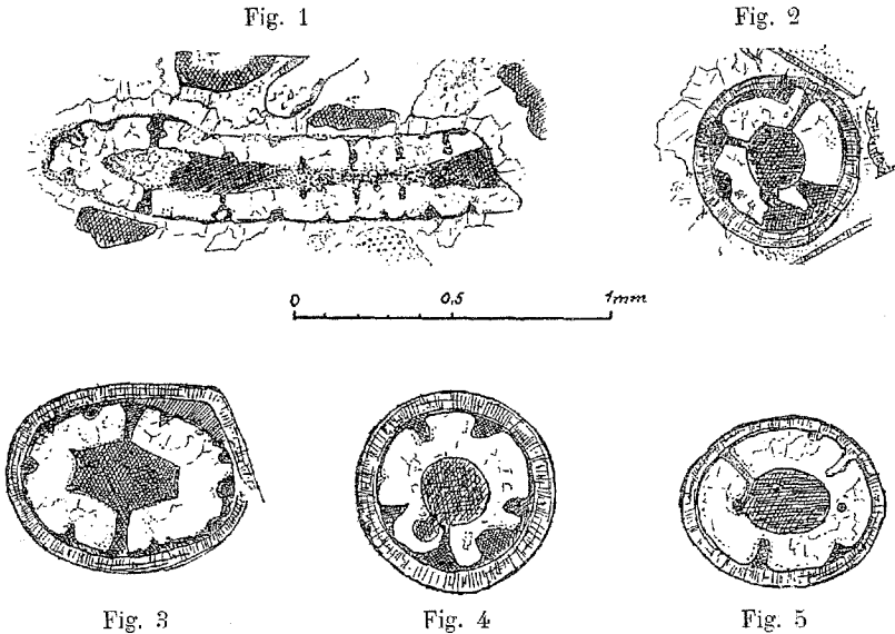
Diplopora Mühlbergi Lorenz aus dem untern Schrattenkalk beim Wildkirchli (Säntisgebiet).
